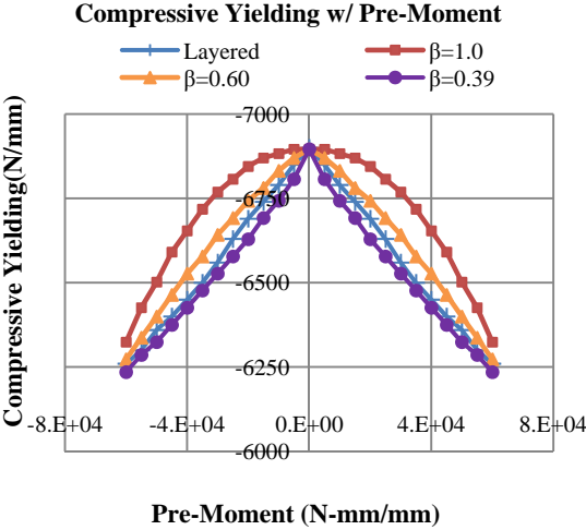
(d) Compressive Yielding on Pre-Moment
